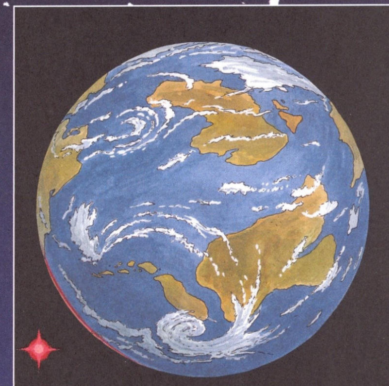
Une des premières photos de la planète "Antarès". En bas, à gauche, l'étoile Antarès. Certaines nuits, elle projette sur la surface de la planète une "lueur" rougeâtre assez intense.
