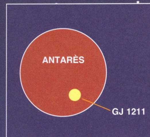
Les étoiles Antarès et GJ 1211 vues de la Terre.
